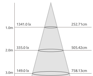
WPR-4B40 Luminance
